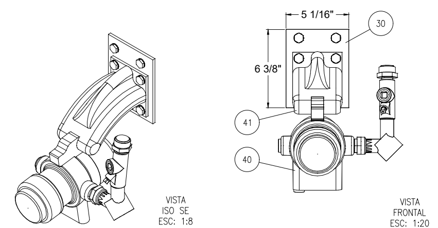
DETECTOR EN CUARTO DE CROMATÓGRAFO
